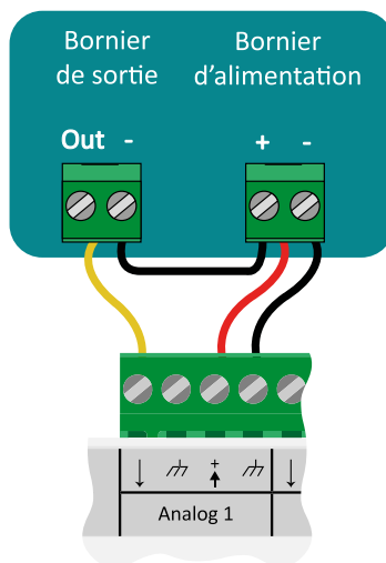
Câblage d'un capteur 0-10V ou 4-20mA en 3 fils
