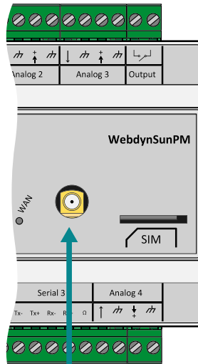
Connecteur SMA
